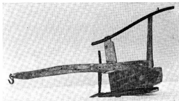
Fig. 42. Potetplog frå Skådel av Syre i Skudenes.
