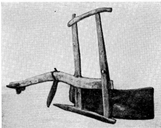
Fig. 10. Plogen frå Brekke i Tysvær, frå andre sida.
