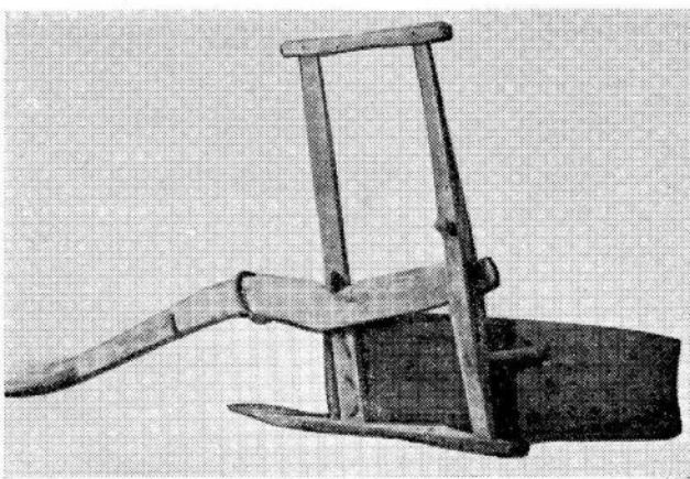
Fig. 2. Plogen frå Haugo i Torvastad frå andre sida.
