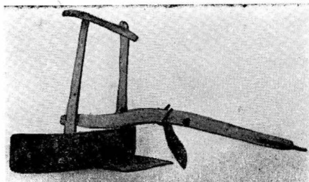
Fig. 9. Plog frå Brekke i Tysvær.
