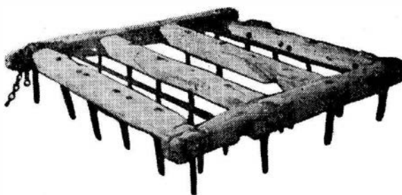
Fig. 24. Horv med jarntindar fra Skeiseid i Fjordesfjorden.
