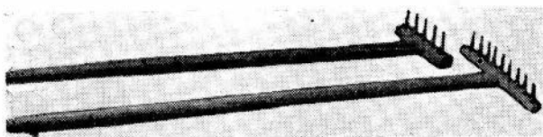
Fig. 30. a. Potetriva frå Øvrabø i Torvastad. b. Mylderiva frå Øvrabø i Torvastad.
