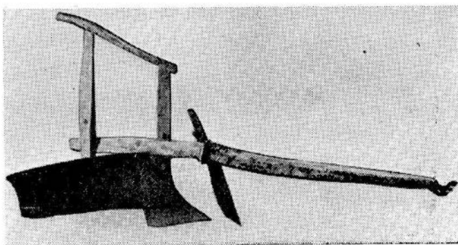
Fig. 15. Plog frå Steinsnes i Skåre.
