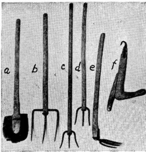
Fig. 26. a. Åkerspade frå Øvrabø, Torvastad. b. Jarngreip frå Øvrabø, Torvastad. c. Breidsletjuga frå Øvrabø, Torvastad. d. Breidsletjuga frå Øvrabø, Torvastad. e. Orgravingsgrev frå Øvrabø, Torvastad. f. Horvekrok frå Øvrabø, Torvastad.
